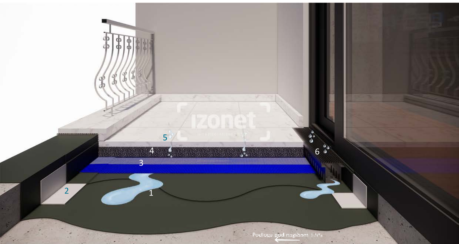
1. ARDEX 8+9 hidroizolacija 2. ARDEX SK 12 traka 3. AQUADRAIN® EK drenažni sloj 4. ARDEX A10 + ARDEX QUARKIES ME granulacije 3.0 - 5.6 mm 5. keramičko/kameno završno popločanje 6. AQUADRAIN FLEX linijski slivnik
